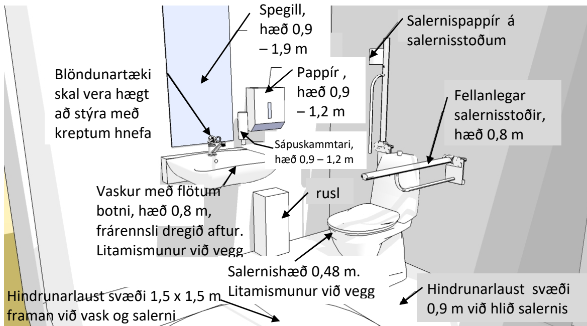
Mynd 5. Dæmi um staðsetningu búnaðar og tækja í baðherbergjum sem innréttuð eru fyrir fólk með hreyfihömlun. Öll mál í metrum
