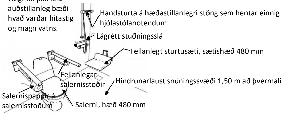
Mynd 6. Dæmi um snyrtingu með sturtusvæði innréttuð fyrir fólk með hreyfihömlun
