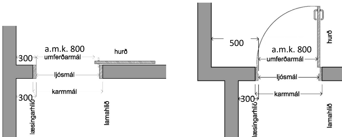
Mynd 1. Hindrunarlaust umferðarmál rennihurðar frístundahúsa sem hönnuð eru á grundvelli algildrar hönnunar. Öll mál í mm
